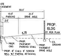
SECTION A-A N.T.S.
