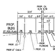
SECTION C-C N.T.S.
